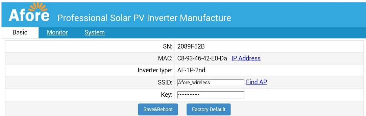
Figuur 2: Instellingen pagina van de omvormer.
